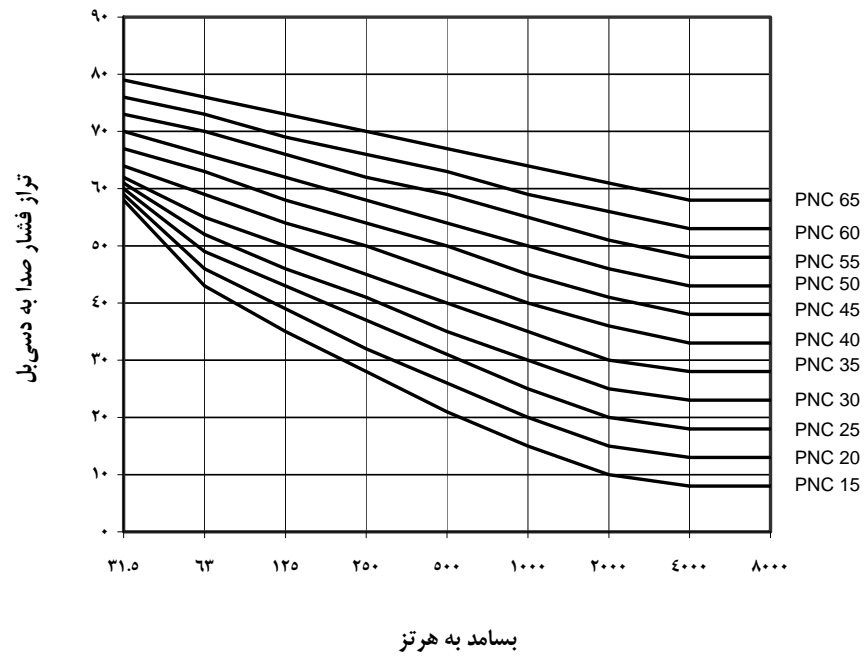
شکل ۱۸-۳-۵: نمودارهای برسنج ترجیحی نوفه PNC
